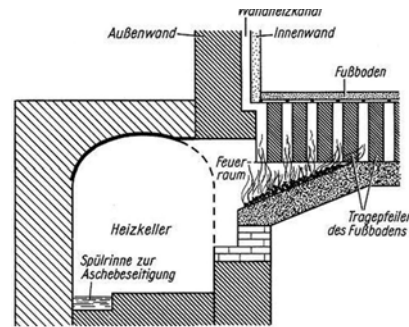
Bild 2 – Schematische Darstellung eines antiken römischen Hypokaustums (Fußboden- und Wandheizsystem)
