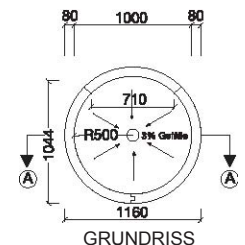
GRUNDRISS
