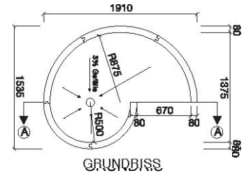
GRUNDRISS
