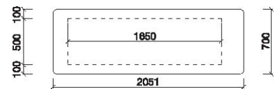
GRUNDRISS
